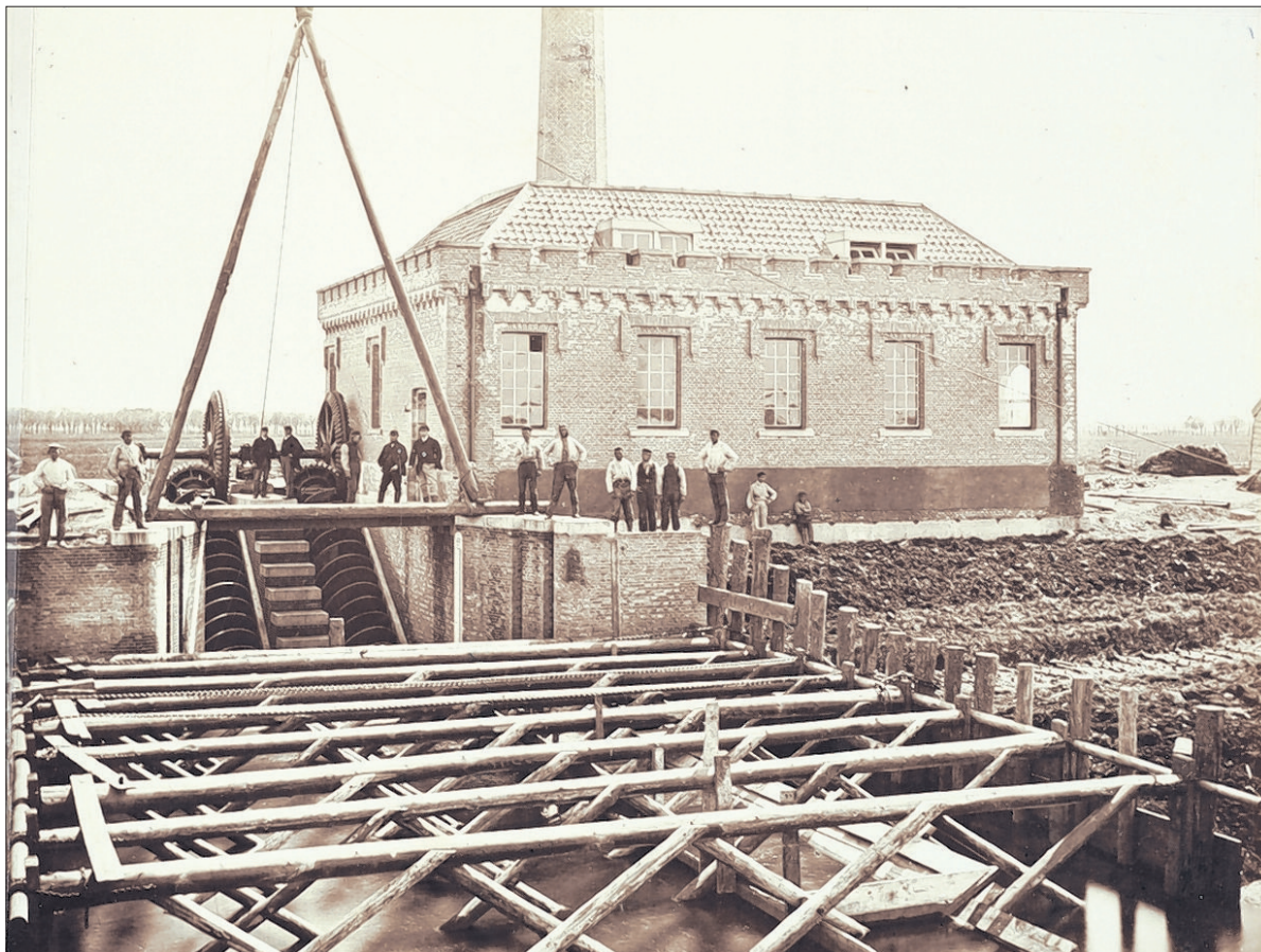
Het Capelse stoomgemaal Jan Anne Beijerinck in aanbouw in 1868. FOTO HOOGHEEMRAADSCHAP SCHIELAND
